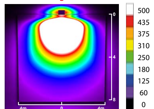
Ausladung 1500mm
