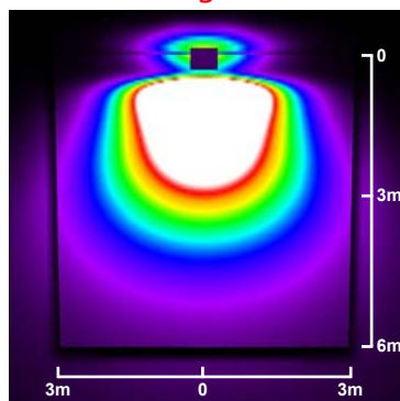
Ausladung 1000mm
